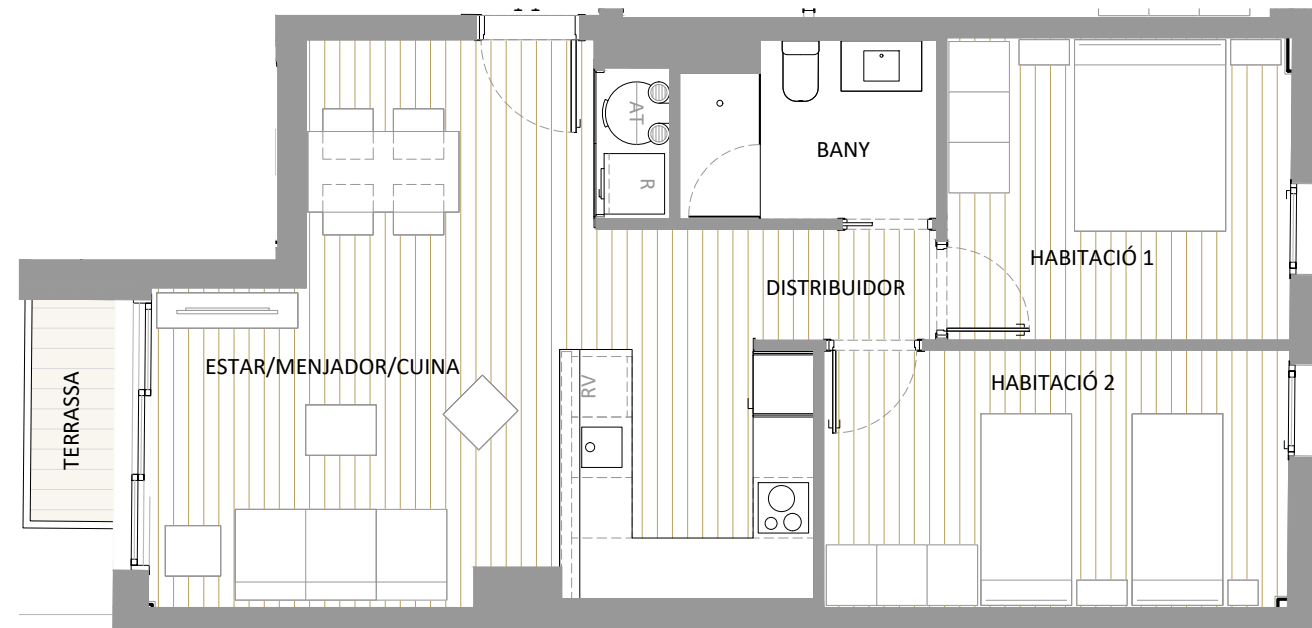
PLANTA PRIMERA
