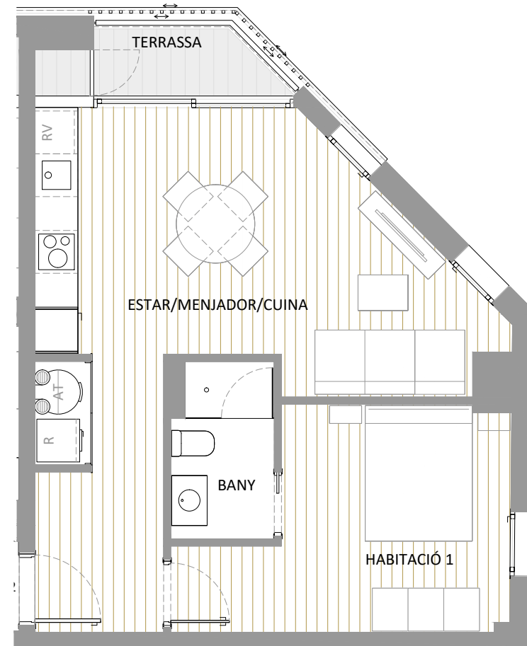
PLANTA PRIMERA
