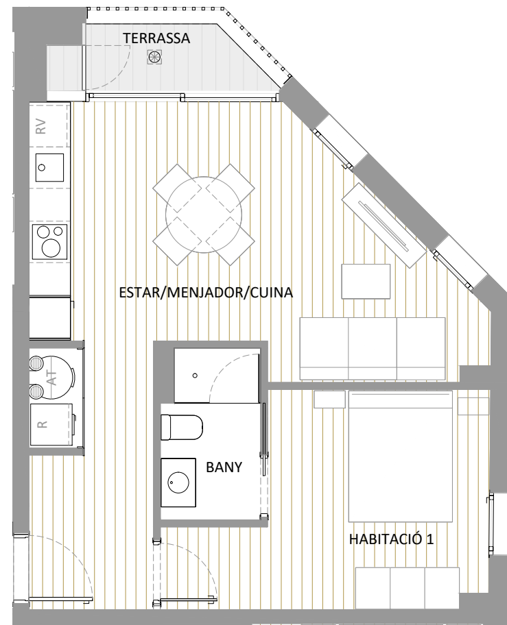
PLANTA BAIXA
