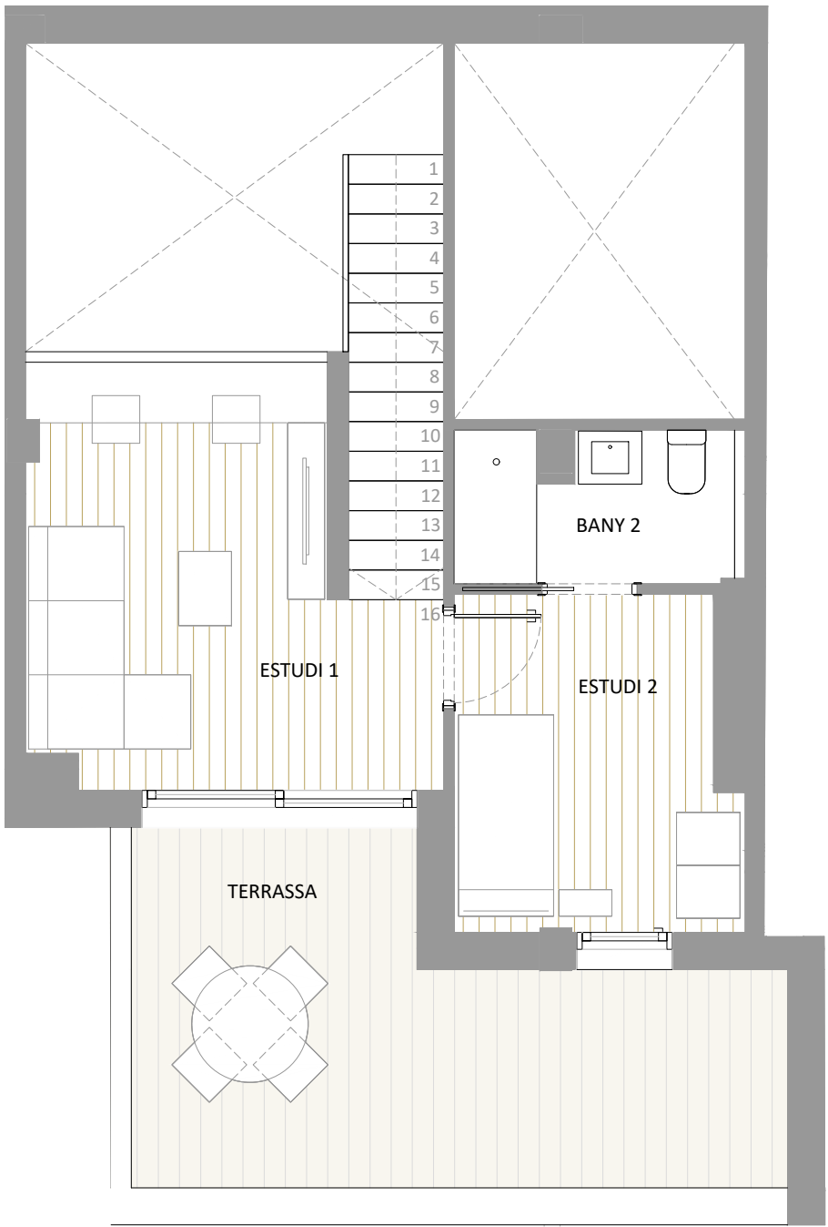
PLANTA SOTA COBERTA
