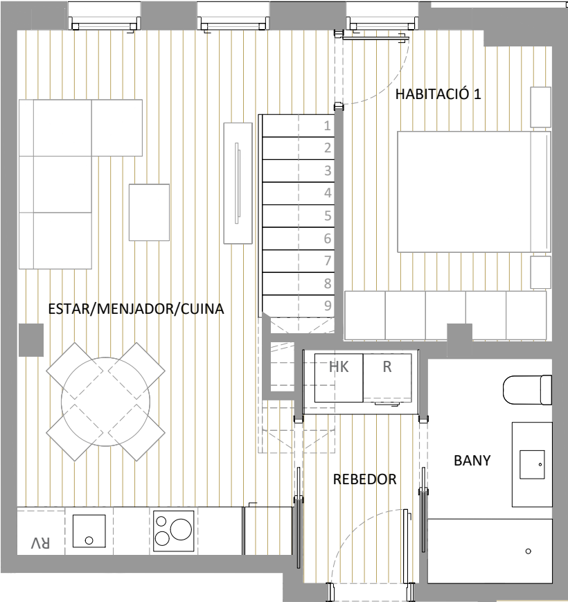
PLANTA SEGONA
