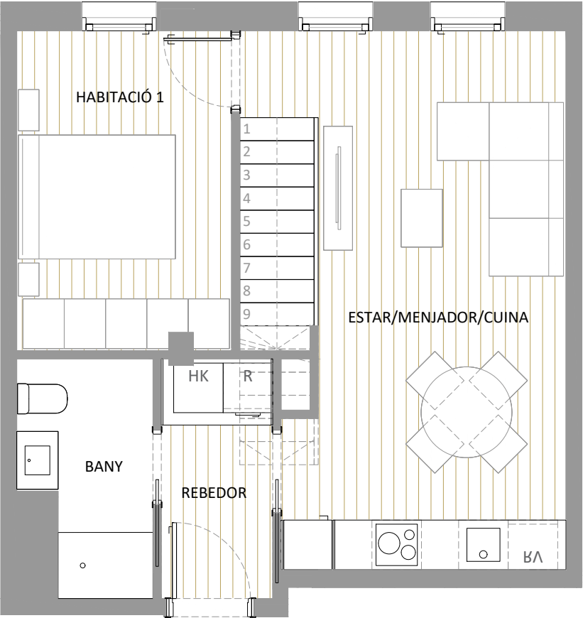
PLANTA SEGONA
