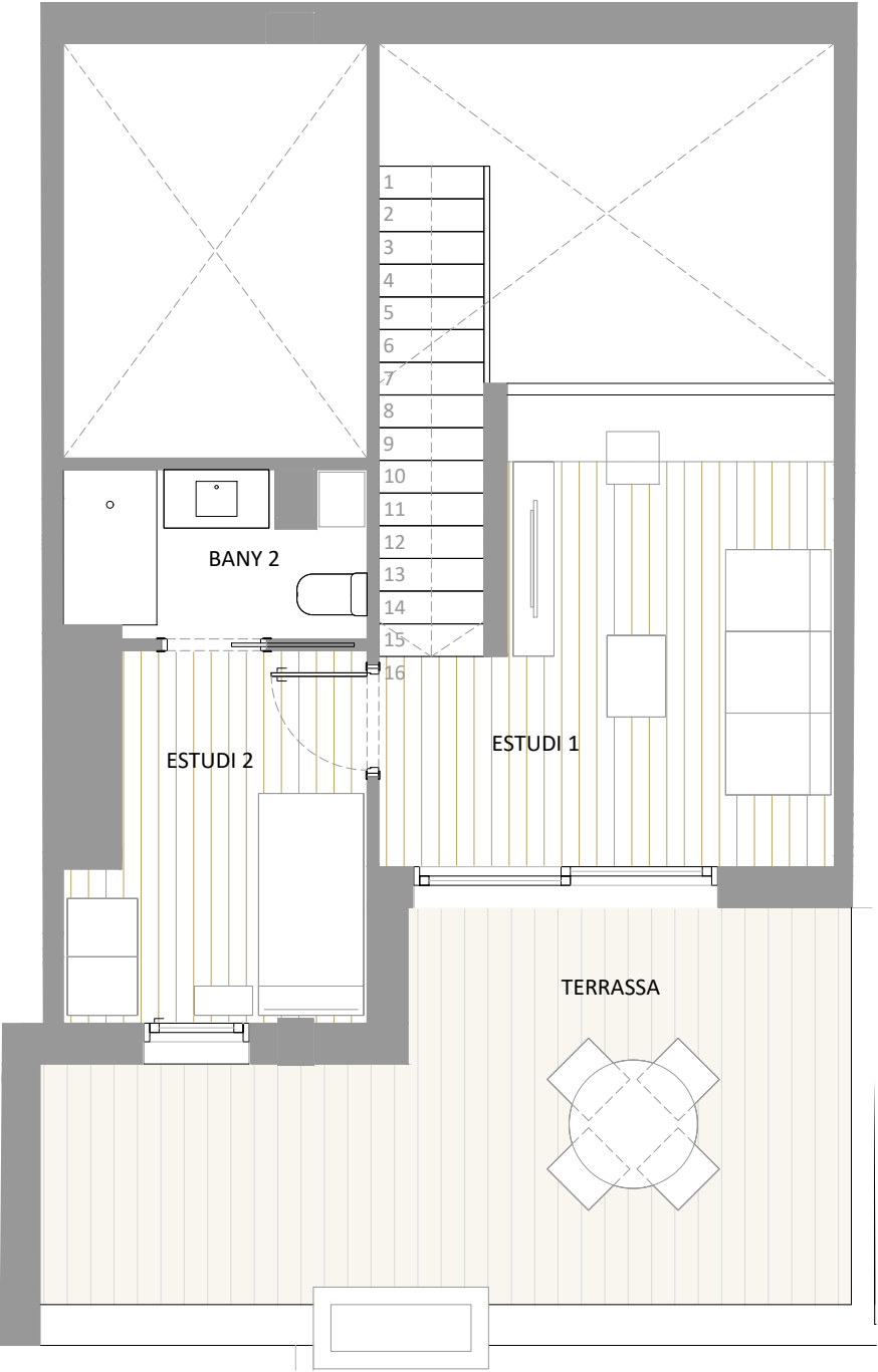
PLANTA SOTA COBERTA
